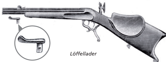
Vertikalblockverschluss
